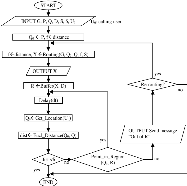
Fig. 4. Guide-me algorithm
